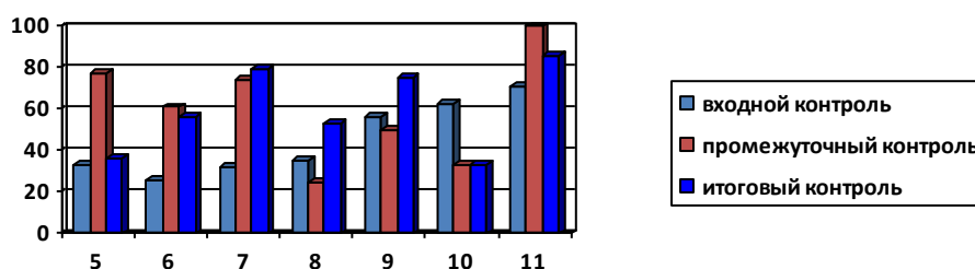
Диаграмма 3
